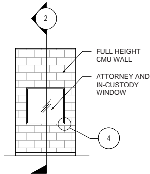
B3 ELEVATION
